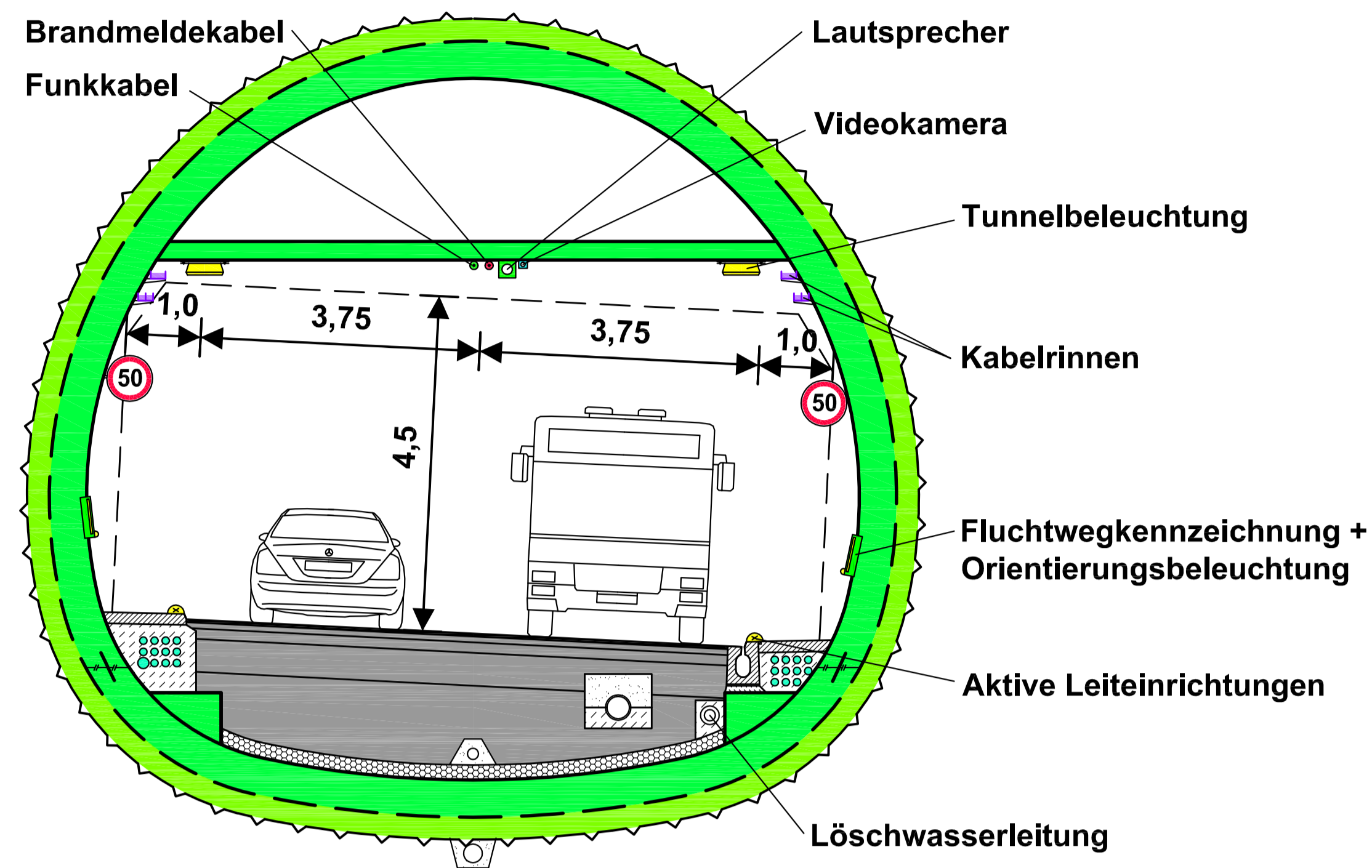
Regelquerschnitt Bergmännische Tunnelröhren
