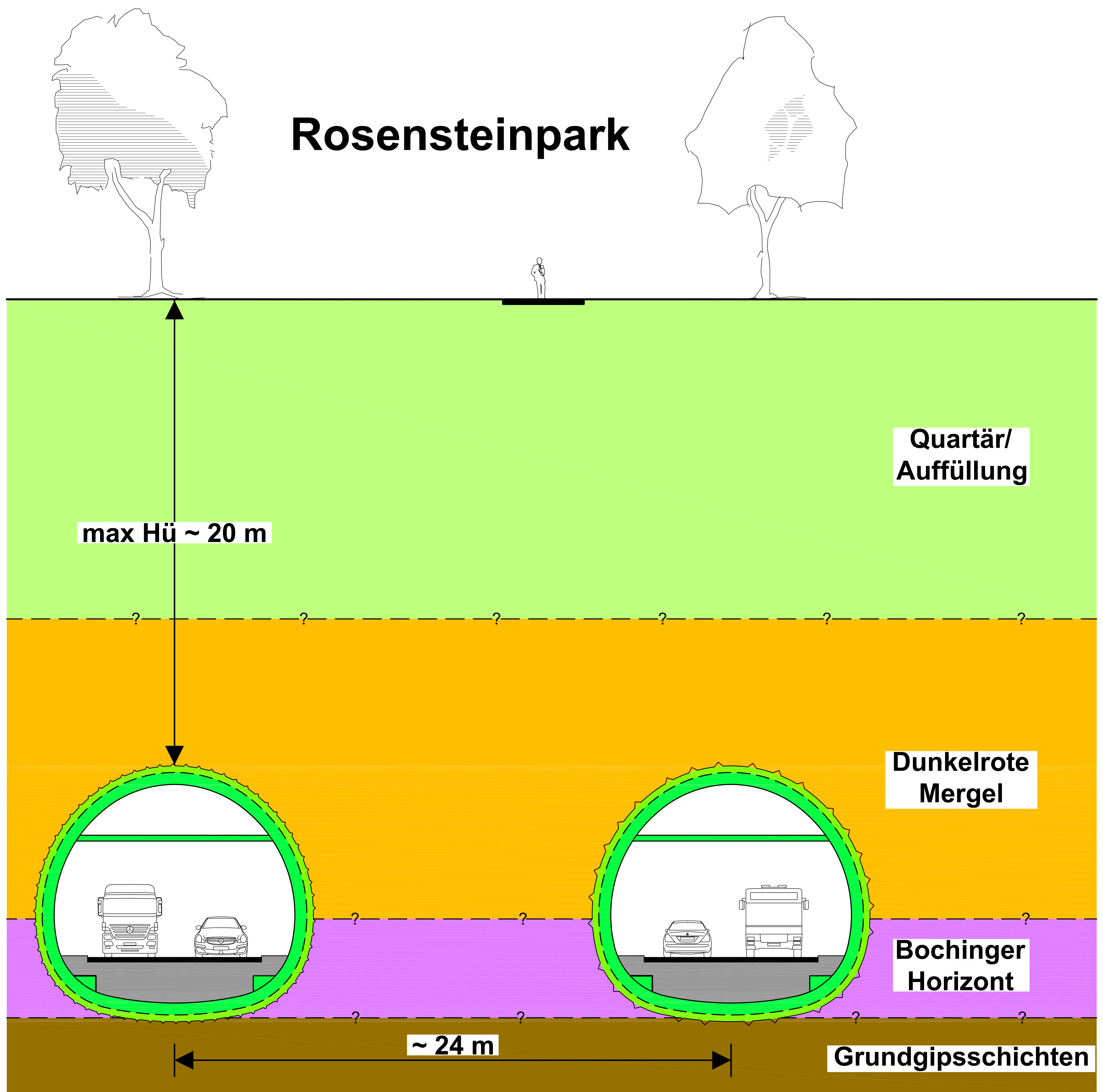
Bergmännische Tunnelröhren im Rosensteinpark - Querschnitt -
